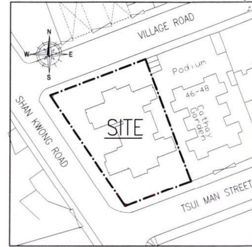
BLOCK PLAN (SCALE : 1 : 1000)
