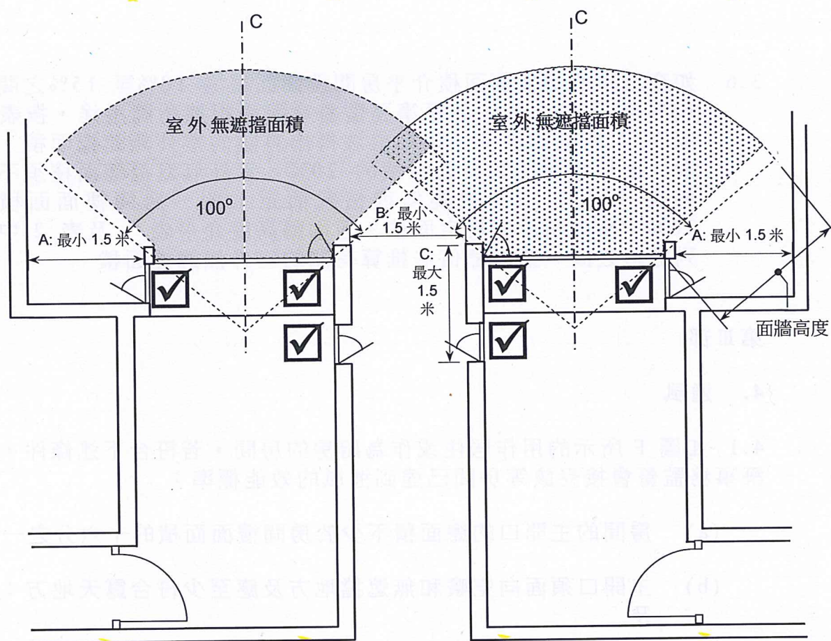
圖 F : 可開啟的通風窗
