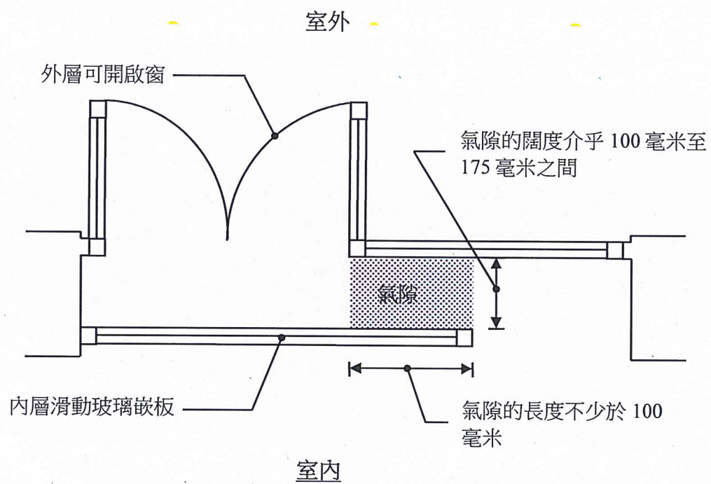
平面圖 (不按比例)
