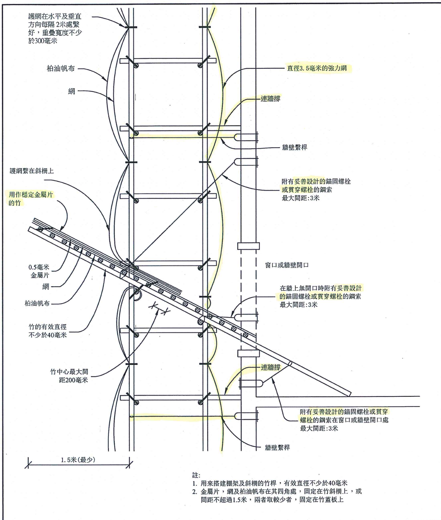
圖3.3 竹斜柵及護網的典型詳圖
