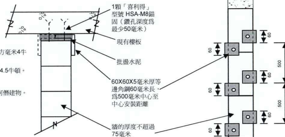
詳圖1
