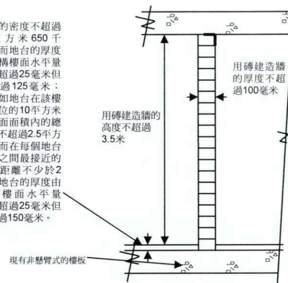
切面圖'A-A'
