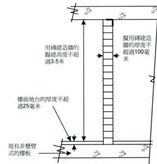
切面圖'A-A'
