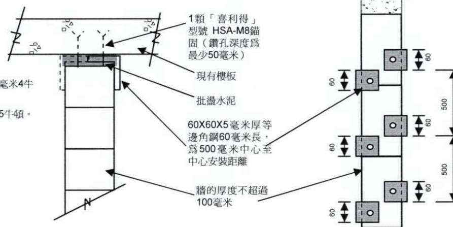
詳圖1
