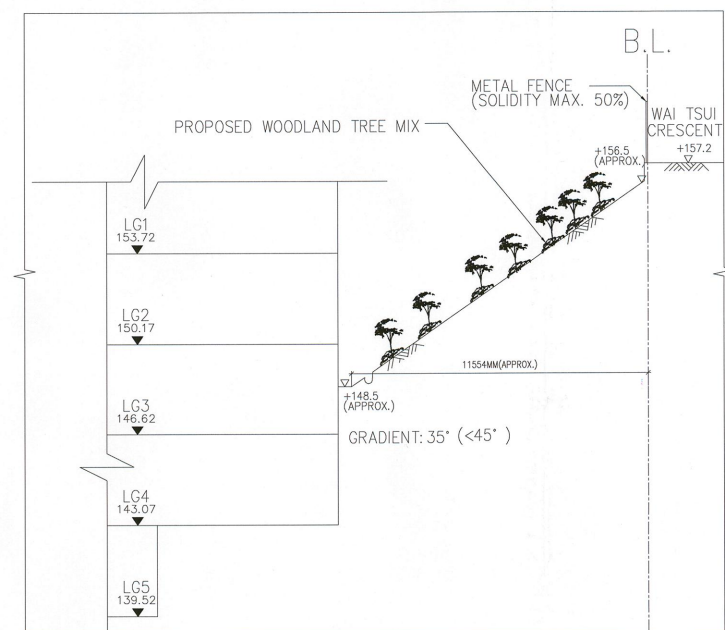
SECTION T-T 1:150
