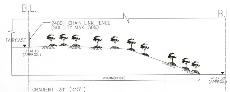
SECTION S-S 1:150
