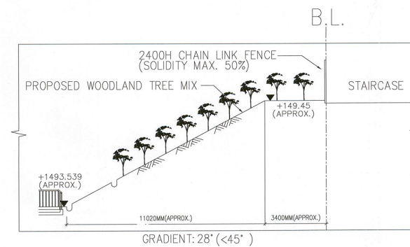
SECTION W-W 1:150
