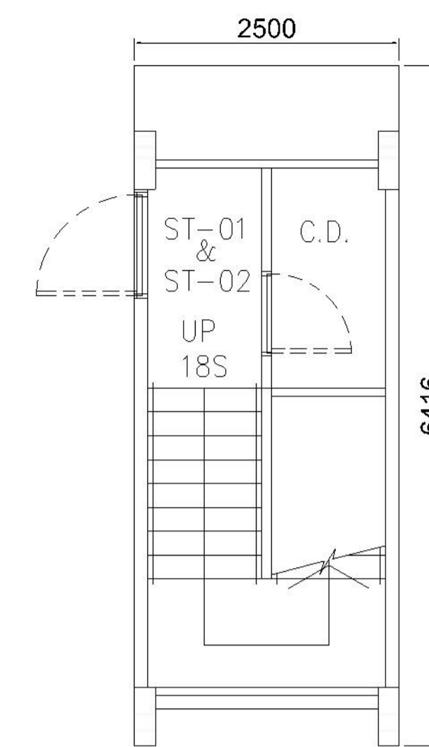
MODULE PLAN MODULE NO.: BOX-06
