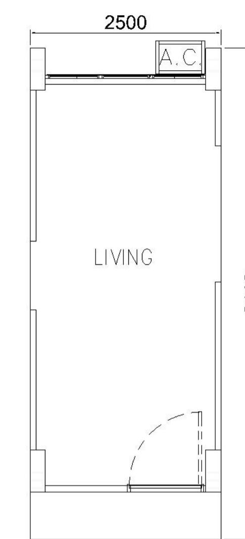
MODULE PLAN MODULE NO.: BOX-05 & BOX-05R
