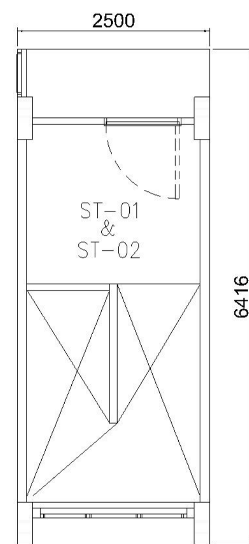
MODULE PLAN MODULE NO.: BOX-06B
