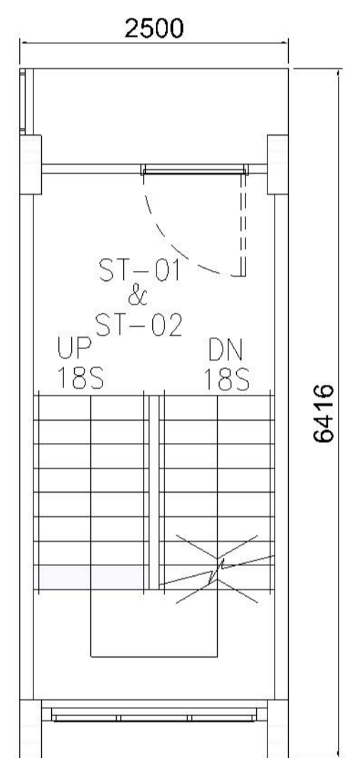
MODULE PLAN MODULE NO.: BOX-06A
