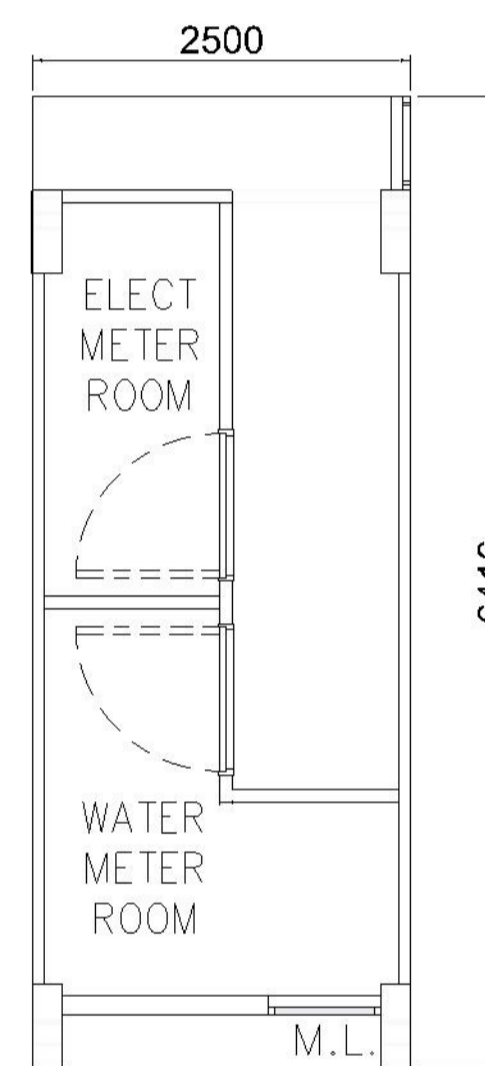
MODULE PLAN MODULE NO.: BOX-07A
