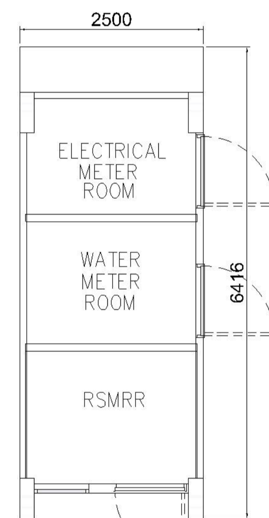
MODULE PLAN MODULE NO.: BOX-07
