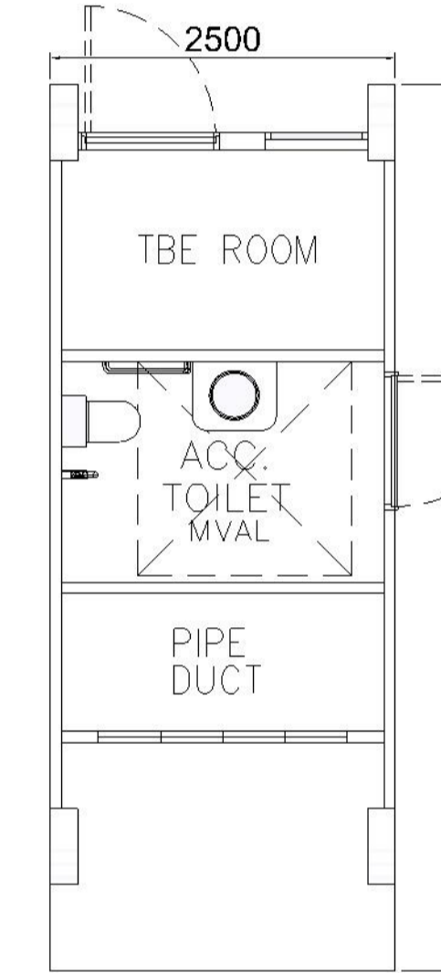
MODULE PLAN MODULE NO.: BOX-11
