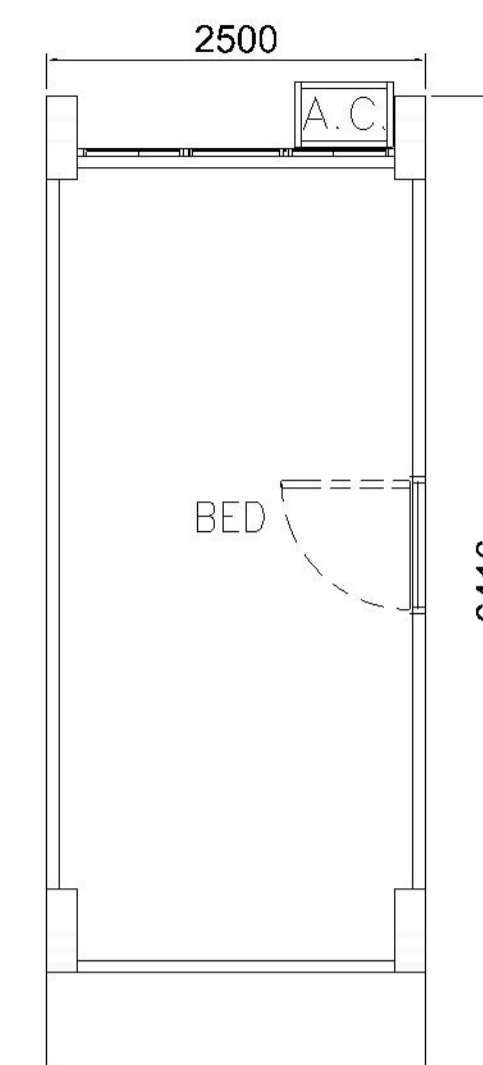
MODULE PLAN MODULE NO.: BOX-04 & BOX-04R
