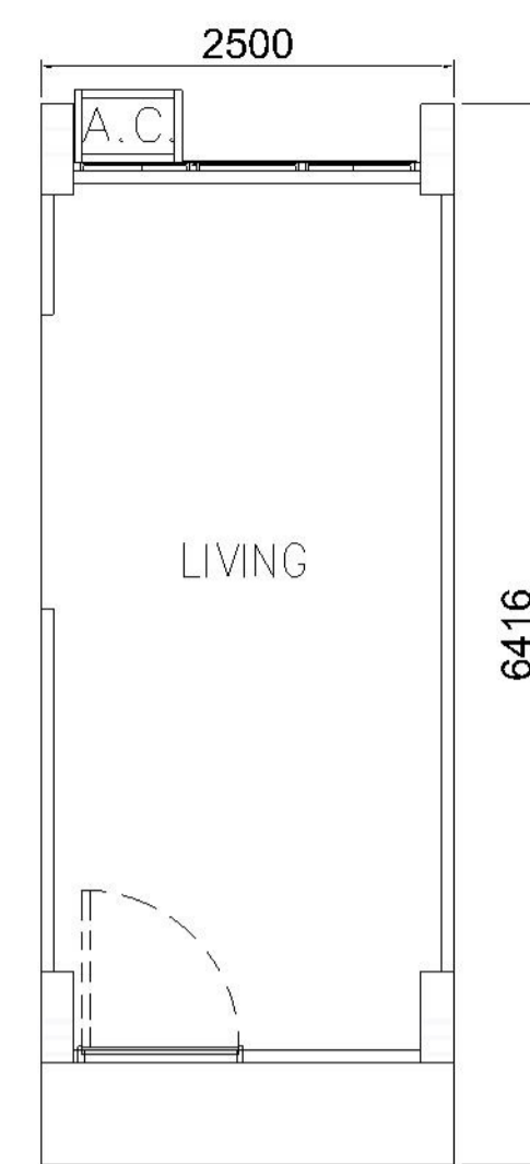
MODULE PLAN MODULE NO.: BOX-03 & BOX-03R
