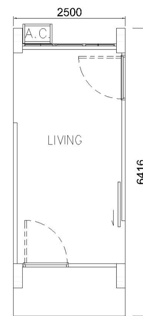
MODULE PLAN MODULE NO.: BOX-09
