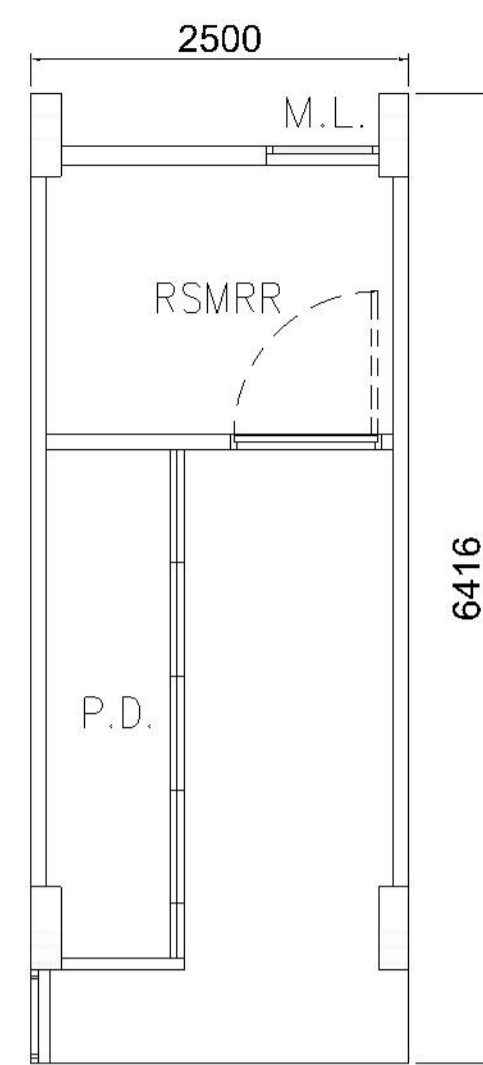
MODULE PLAN MODULE NO.: BOX-01A
