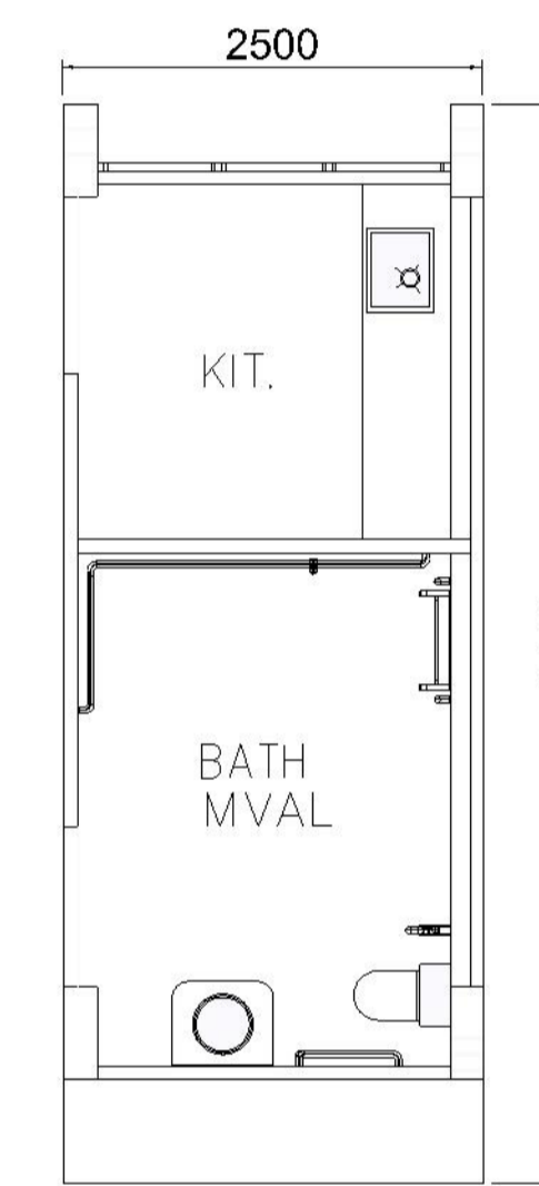
MODULE PLAN MODULE NO.: BOX-10
