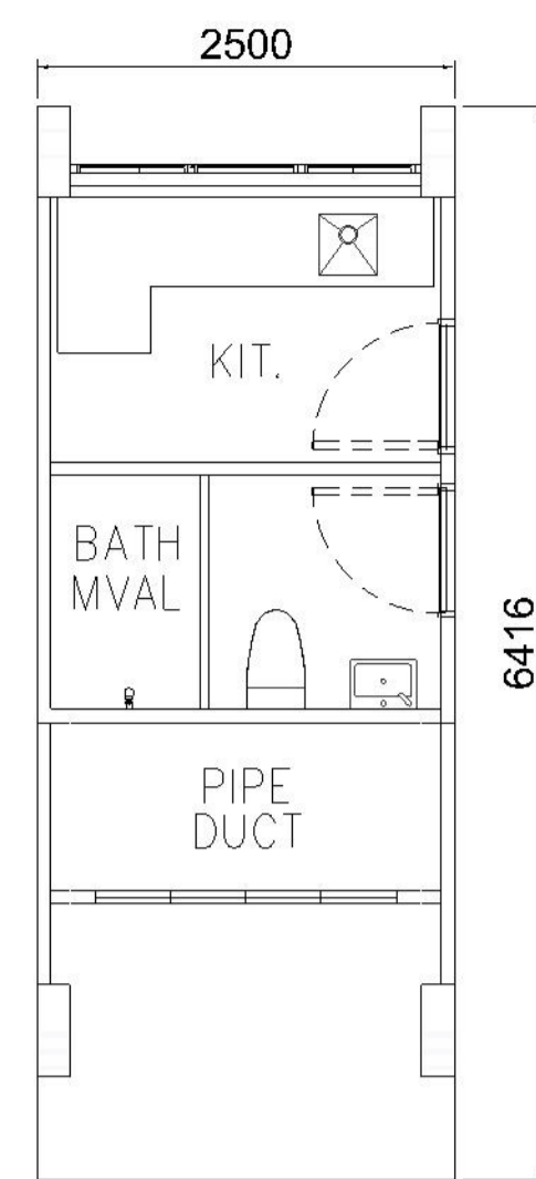
MODULE PLAN MODULE NO.: BOX-02 & BOX-02R
