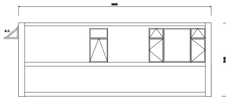
ELEVATION A
