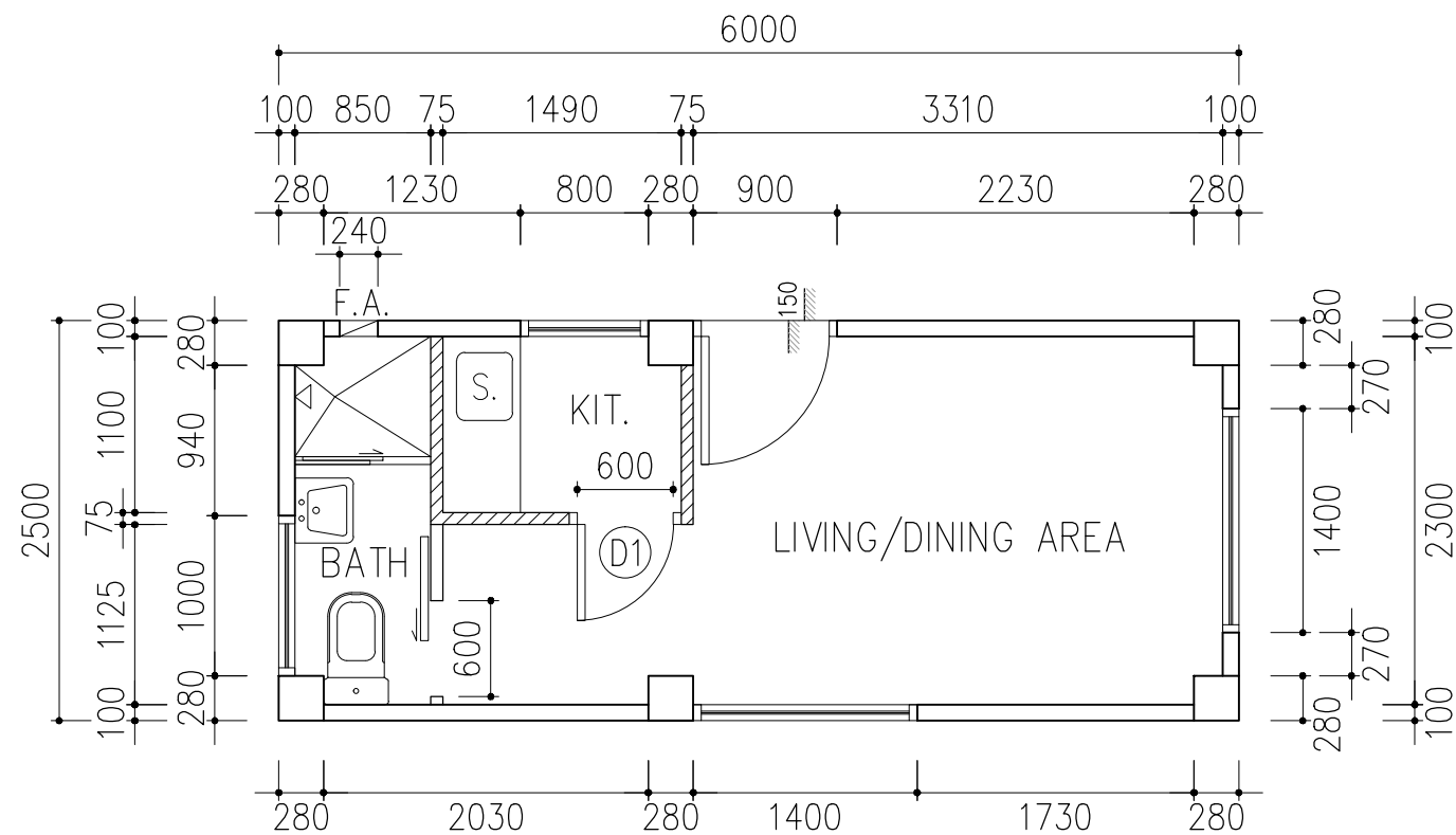
G/F PLAN
