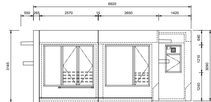
ELEVATION B
