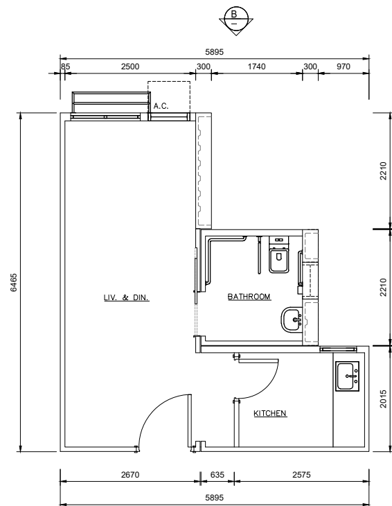
MiC MODULE UNIT D TYPE D1, D2, D3
