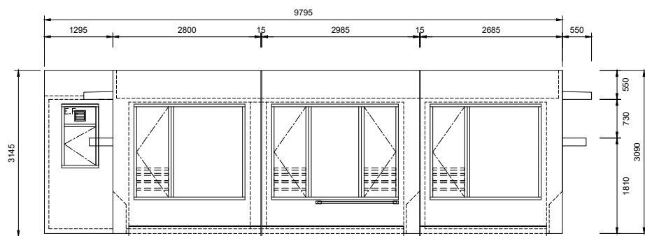
ELEVATION B
