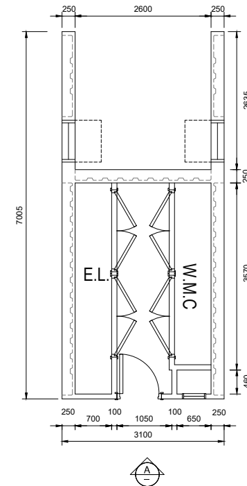
MiC MODULE EMR TYPE E1
