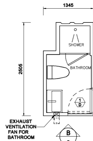
PLAN Module No. YLW-T02 Module No. (YLW-T02R) MIRRORED
