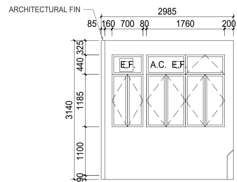
ELEVATION A
