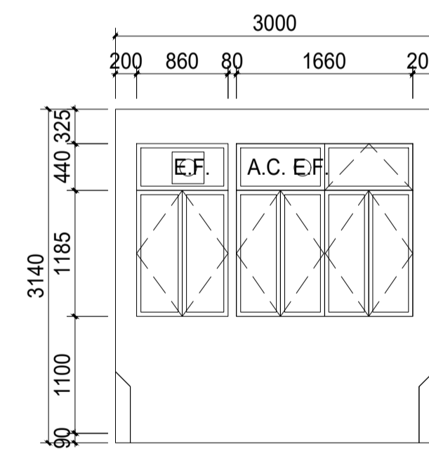
ELEVATION A
